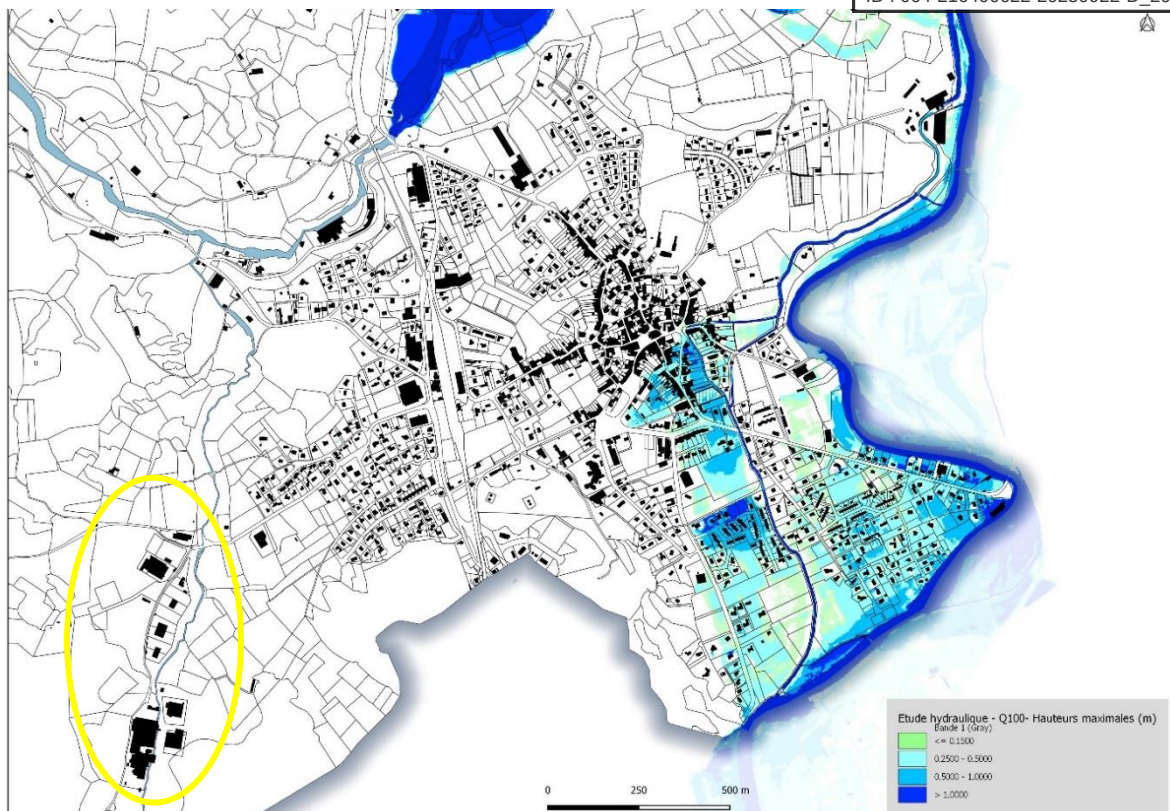
Figure 25- Etude hydraulique réalisé à l'échelle de la CCVO autour du Gave d'Ossau 2021/2023
