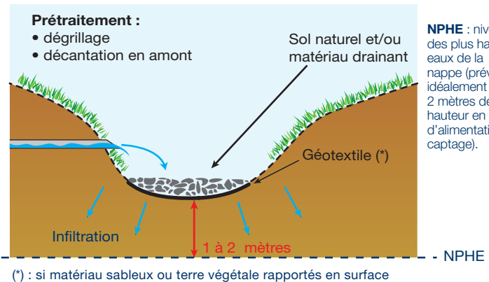
Schéma type (bassin sec)
