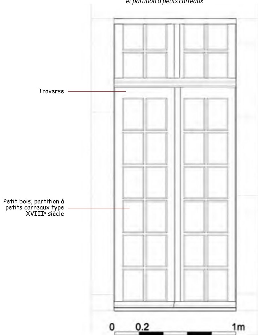
Fenêtre XVIII e siècle à traverse et partition à petits carreaux
