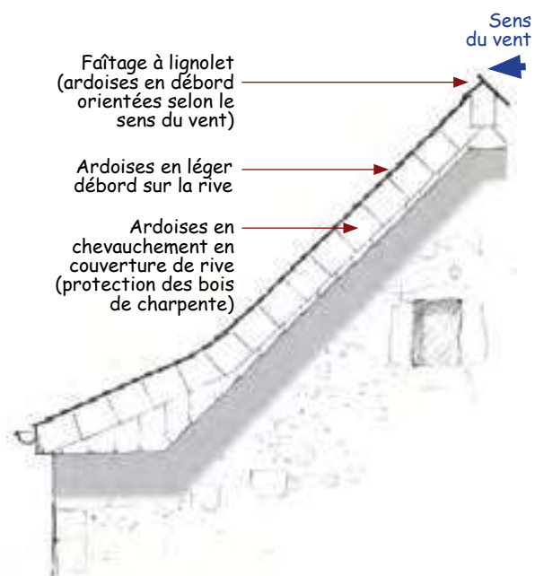
Détail d'une rive en ardoise
