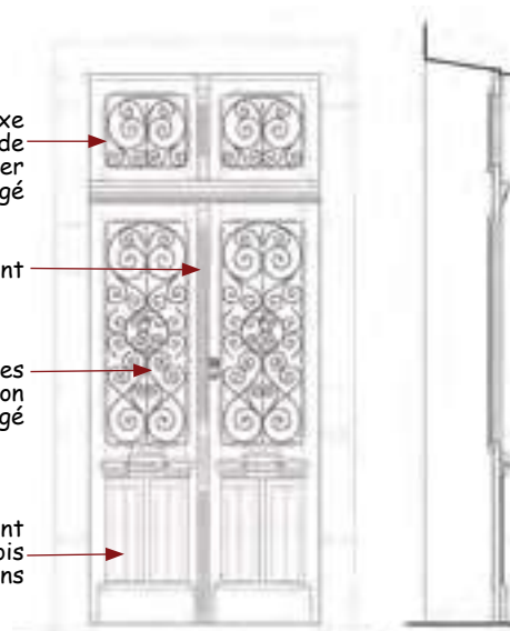
Porte type XX e siècle, vantail double, menuiserie et vitrage, imposte, grilles de protection en ferronnerie.
