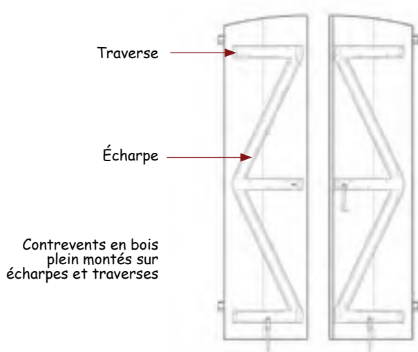
Face interne
