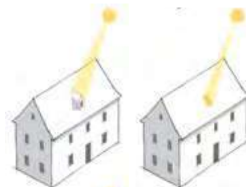
La lucarne traditionnelle avec sa toiture couvrante présente l'avantage de protéger le toit des excès du rayonnement solaire zénithal en été et limite la surchauffe du comble.
