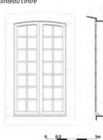
Partition à petits carreaux avec linteau cintré
