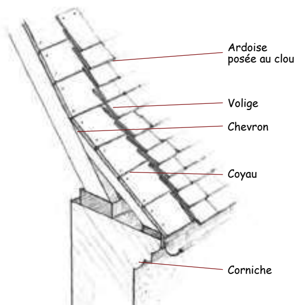
Clouage à 1 clou
