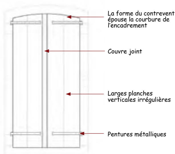
Face externe
