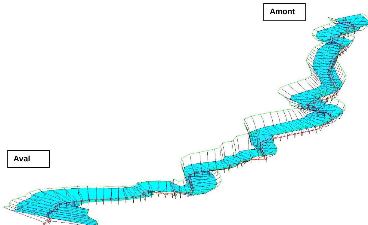
FIG. 11. VISUALISATION DU MAILLAGE DU MODÈLE DE L'AMEZPETU
